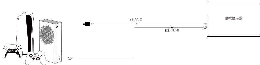
☆HDMI/Type-C端口连接Switch接线示意图
