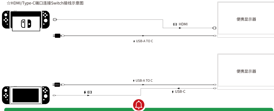
☆HDMI/Type-C端口连接Switch接线示意图
